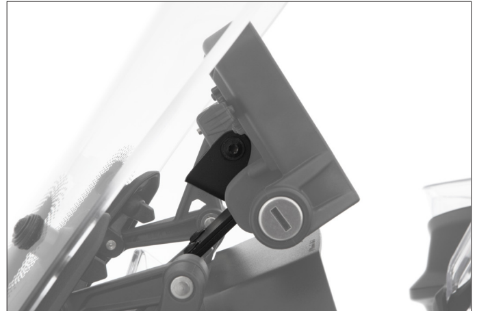
Wunderlich Navihalterung (Art.-Nr.: 21173-002), Befestigung oberhalb des TFT-Kombiinstrumentes
