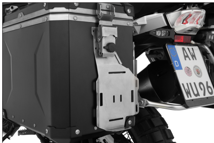
Das Wunderlich Koffer-Rack an der BMW R 1250 GS (Art.-Nr.: 20570-500)
