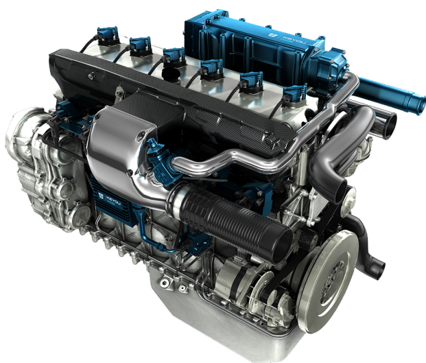
Rendering eines 7.8l Wasserstoffmotors mit KEYOU-inside Technologie.
