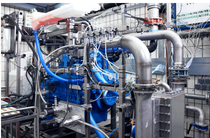
H2-Motor mit KEYOU-inside auf Prüfstand (8l-Motor)
